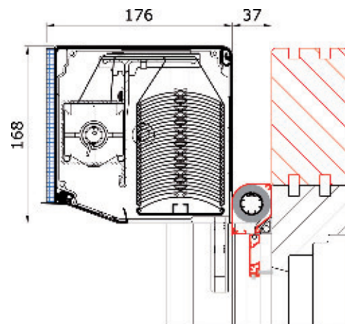
06 MIT INTEGRIERTEM IGI-ROLLO VORO PUTZ Raff-Darstellung Kastengröße 16 mit 80R Lamellen
